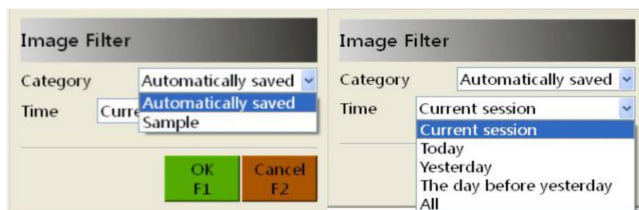
Рис. 6.4 Фильтр изображений
